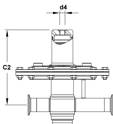
Optional dome-loading
